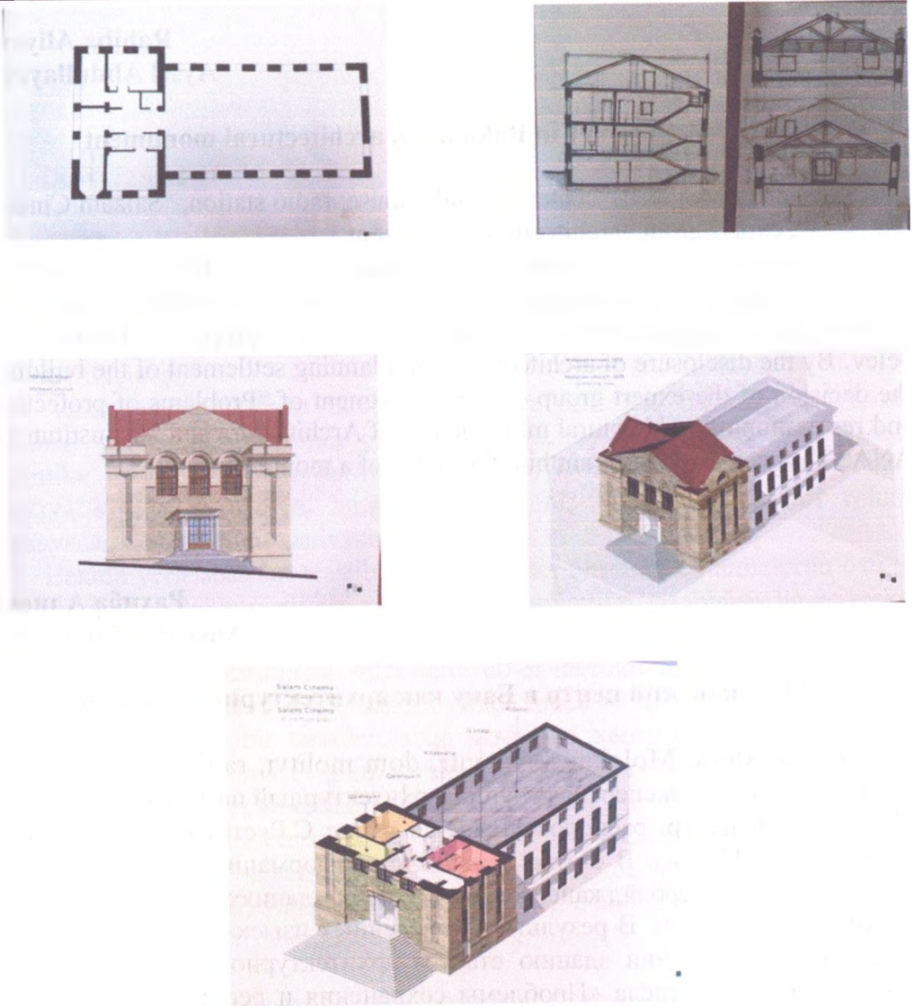
Şəkil 2. Binanın planı, fasad və aksonometrik kəsikləri
