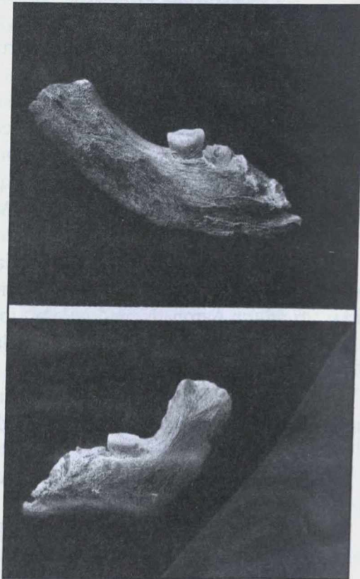
Şəkil 11. Azıxantropun alt çənəsi.
