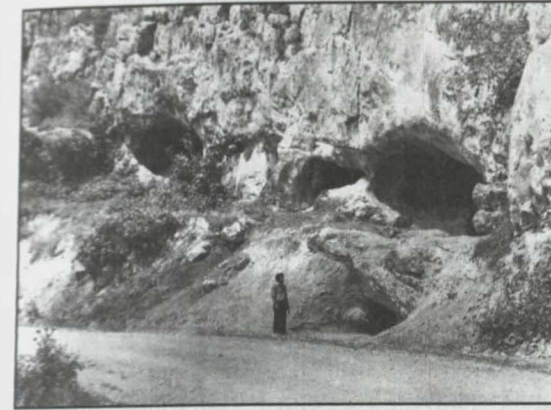
Şəkil 12. Qarabağ. Tağlar paleolit düşərgəsinin ümumi görünüşü
