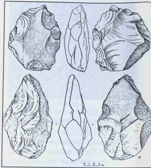
Şəkil 9. Azıx düşərgəsi. Əl çapacaqları. Qədim aşel mədəniyyəti. VI təbəqə
