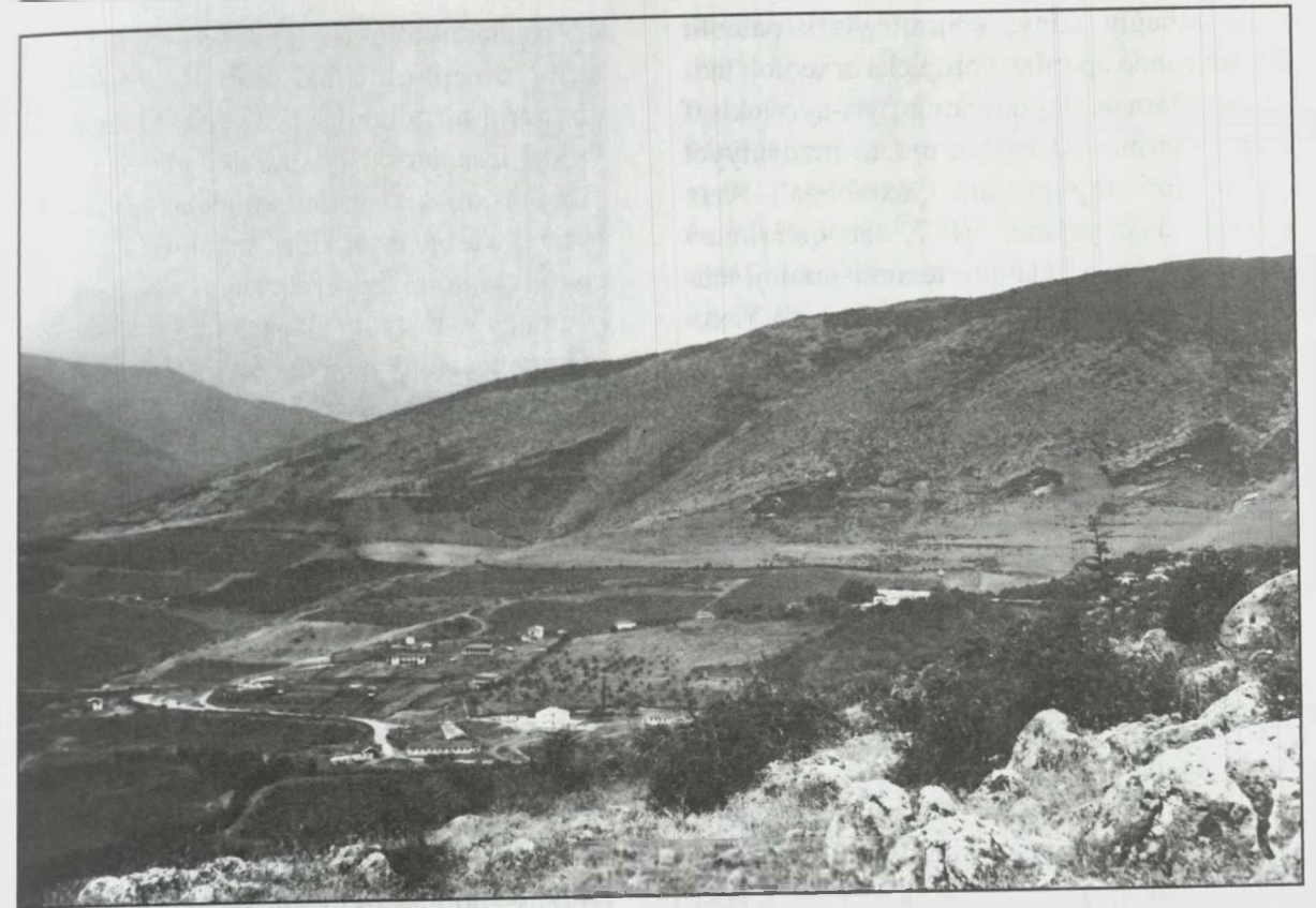
Şəkil 1. Qarabağ Tuğ çökəkliyi
