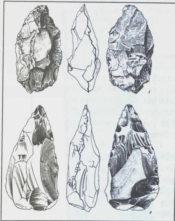
Şəkil 10. Azıx düşərgəsi. Əl çapacaqları. Orta aşel mədəniyyəti. V təbəqə
