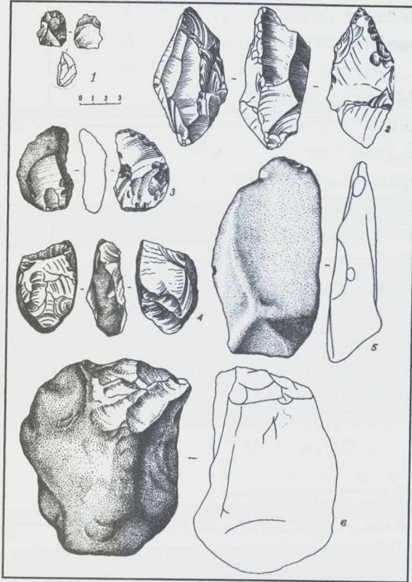
Şəkil 8. Azıx düşərgəsi. Əmək alətləri. Quruçay mədəniyyəti. X təbəqə.
