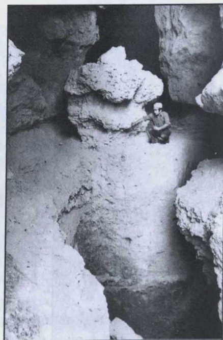
Şəkil 6. Azıx paleolit düşərgəsi aşağı təbəqələrin ümumi görünüşü (VI-X təbəqələr)
