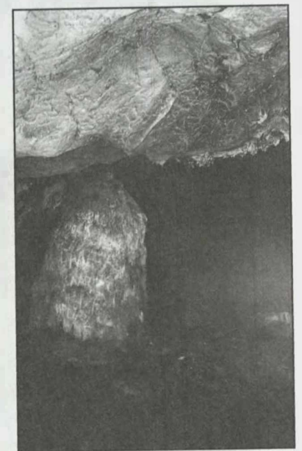
Şəkil 4. Azıx düşərgəsi. Stalaqnat dirək
