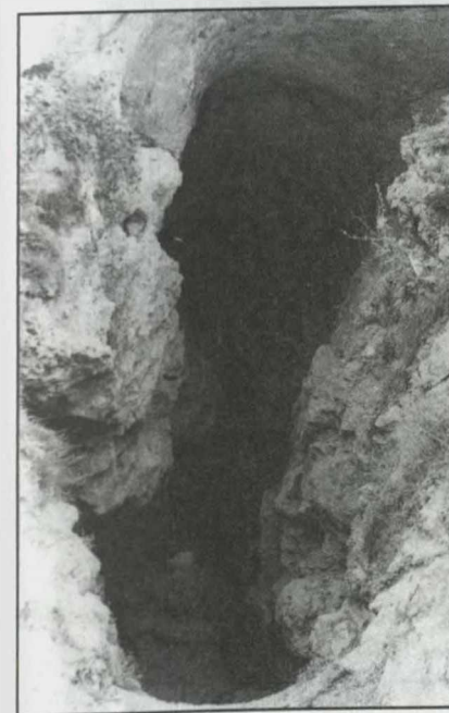
Şəkil 2. Azıx düşərgəsinin giriş yolu
