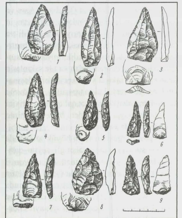
Şəkil 13. Tağlar düşərgəsi. Mustye mədəniyyəti. İtiucullar. IV (a) təbəqə
