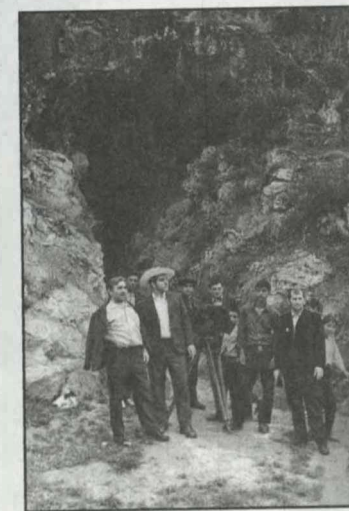
Şəkil 3. Azıx düşərgəsinin ümumi görünüşü. 1975-ci il
